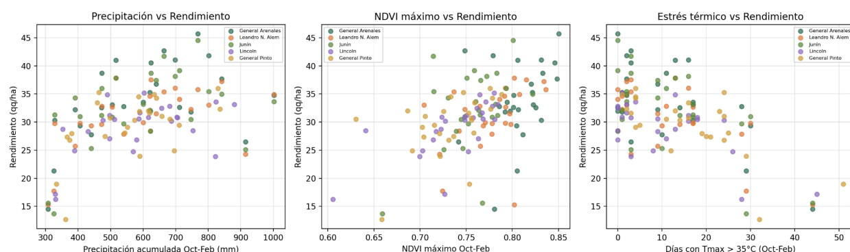
Figura 4. Relación entre variables predictoras clave (ventana octubre-febrero) y rendimiento de soja por partido. Izquierda: precipitación acumulada. Centro: NDVI máximo. Derecha: días con temperatura máxima superior a 35°C. Fuente: elaboración propia.
