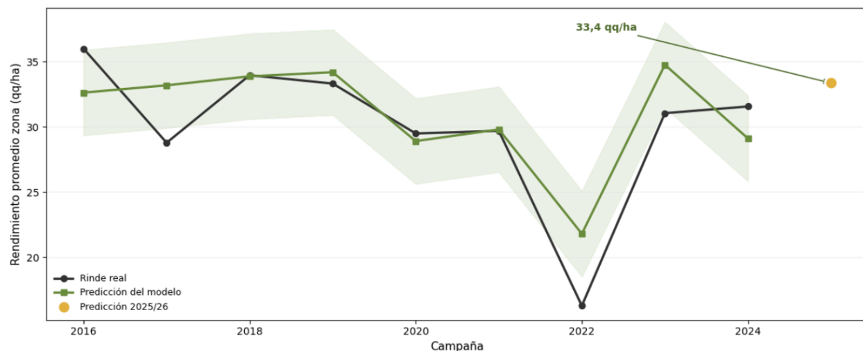
Figura 7. Rendimiento promedio zonal real (línea negra) y predicho por el modelo con datos hasta enero (ventana oct_ene, validación walk-forward; línea verde) para las campañas 2016-2024, junto con la predicción para la campaña 2025/26 (punto dorado, ventana oct_mar). La banda sombreada indica \pm el error medio del modelo. Fuente: elaboración propia.
