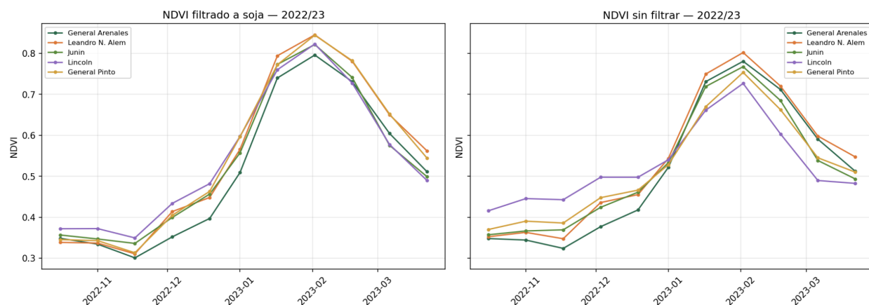
Figura 9. NDVI de la campaña 2022/23 por partido, filtrado a píxeles de soja según el Mapa Nacional de Cultivos del INTA (izquierda) y sin filtrar (derecha). Fuente: elaboración propia a partir de datos MODIS e INTA.
