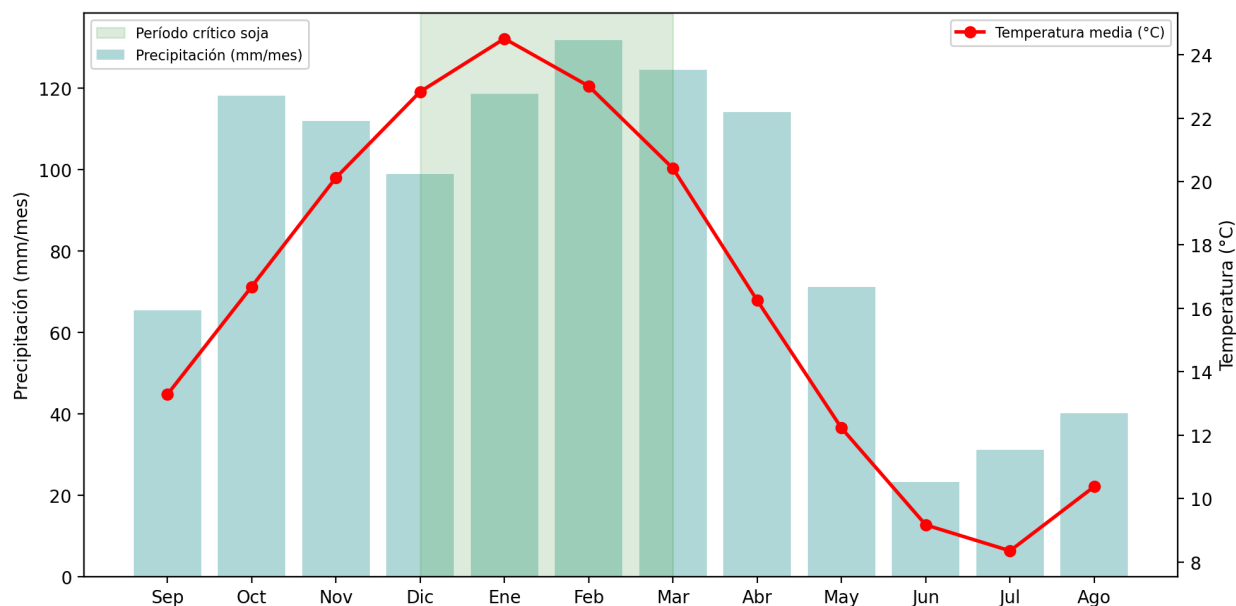
Figura 2. Ciclo anual promedio de temperatura media y precipitación en la zona de estudio (1999-2025). La zona sombreada indica la etapa reproductiva de la soja. Fuente: elaboración propia a partir de datos NASA POWER.
